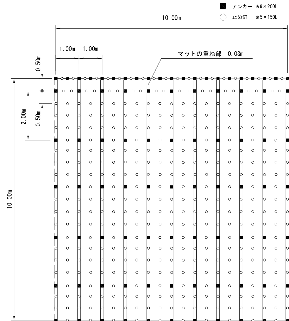
標準展開図
