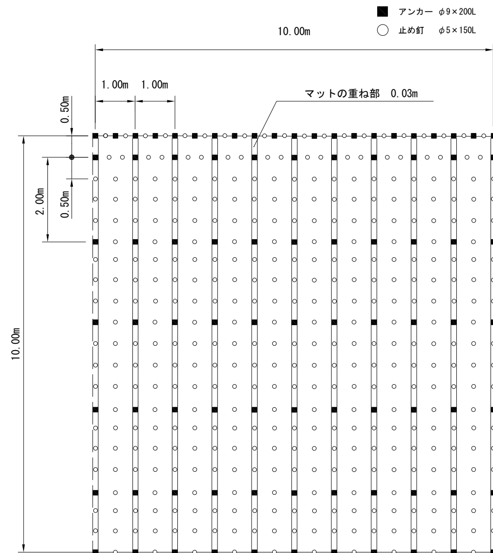
標準展開図
