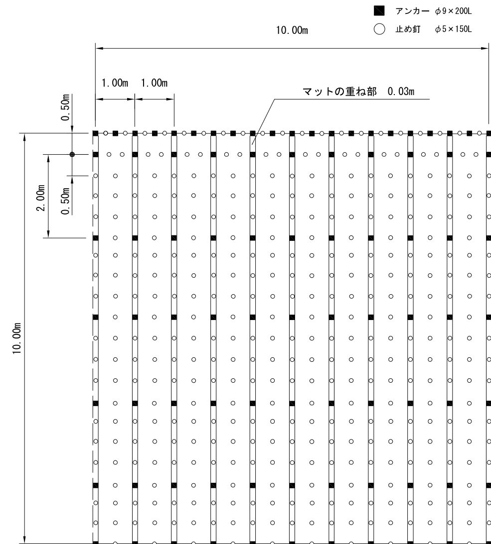
標準展開図
