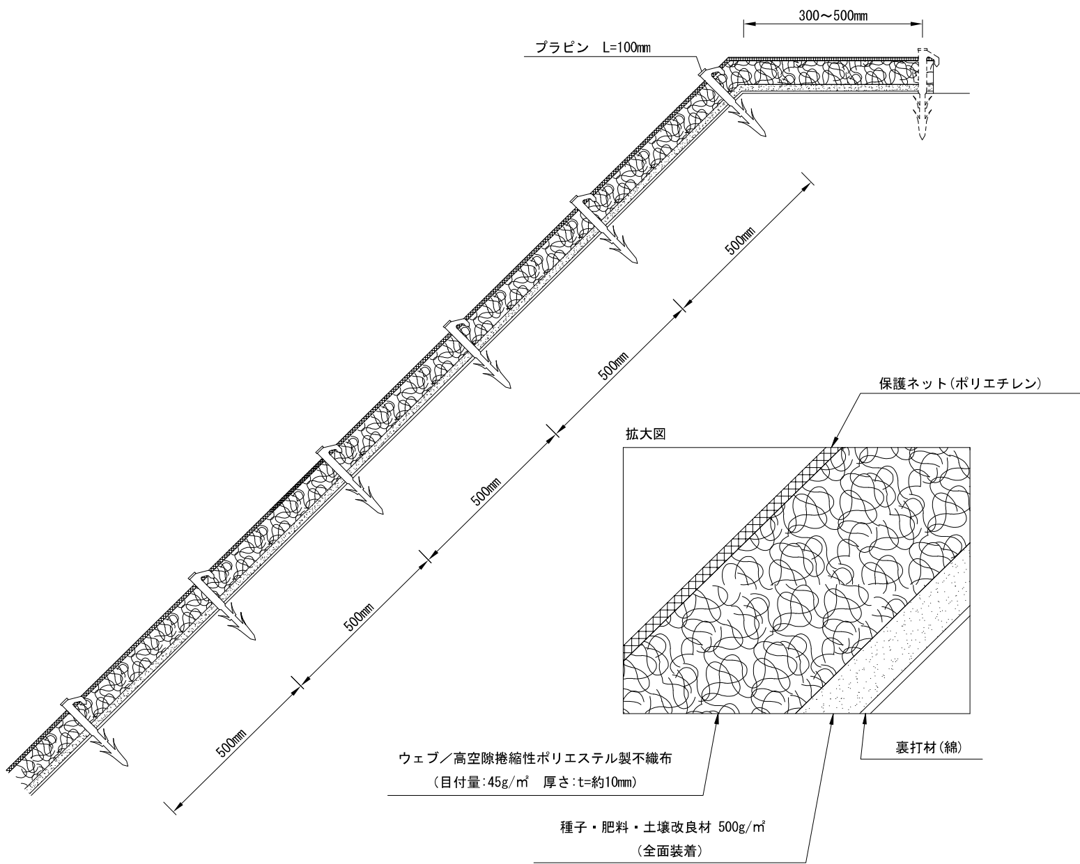
材料表 (100㎡当り)
