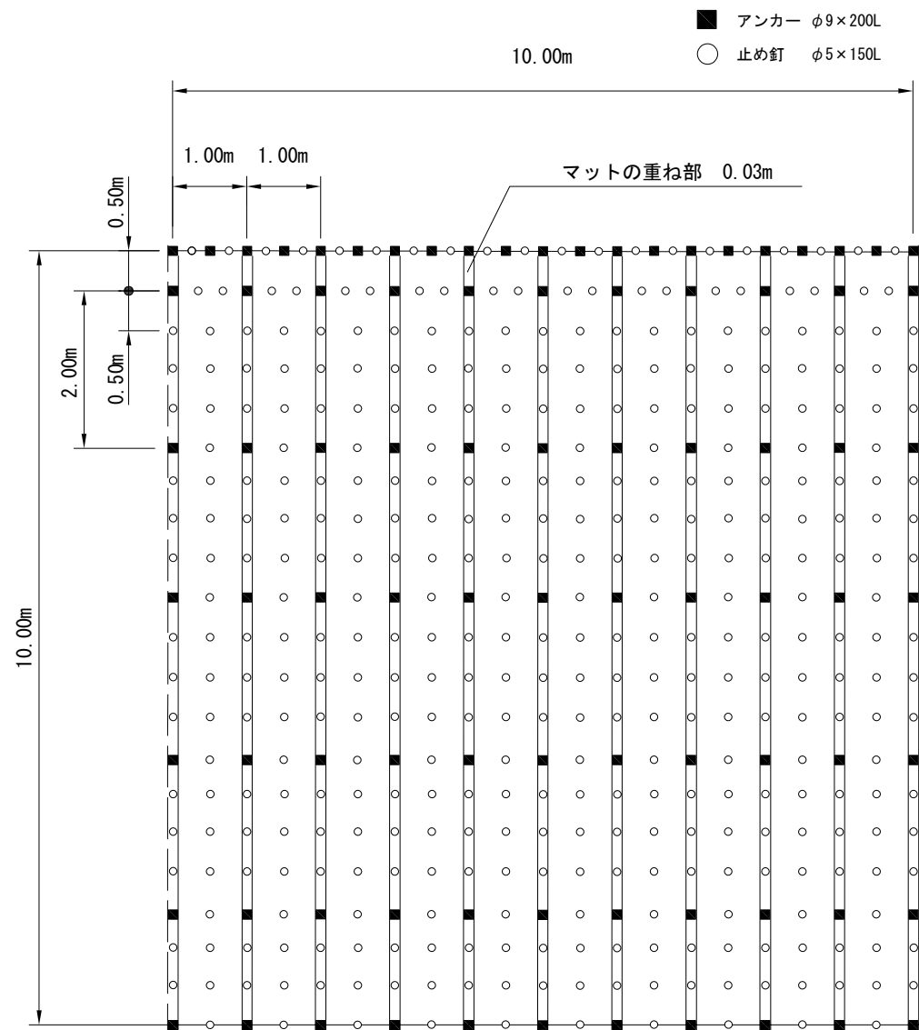
標準展開図
