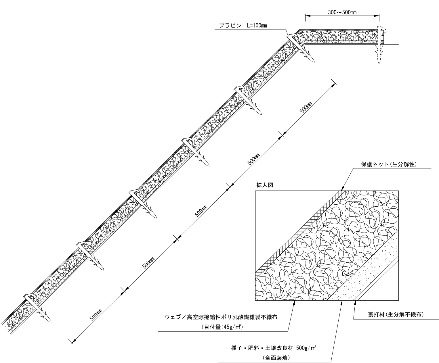
材料表（100㎡当り）
