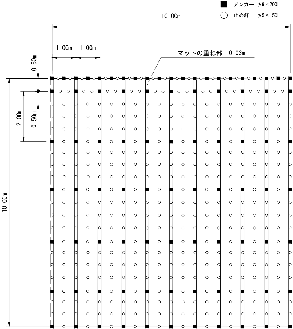
標準展開図
